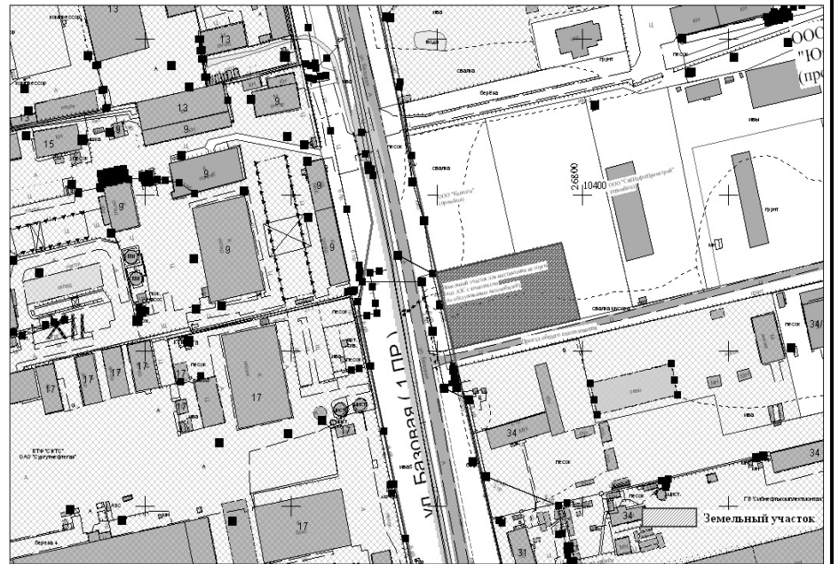
Схема границ земельного участка для строительства АЗС с комплексом по обслуживанию автомобилей в Восточном промрайоне по улице Базовой М 1:2000
